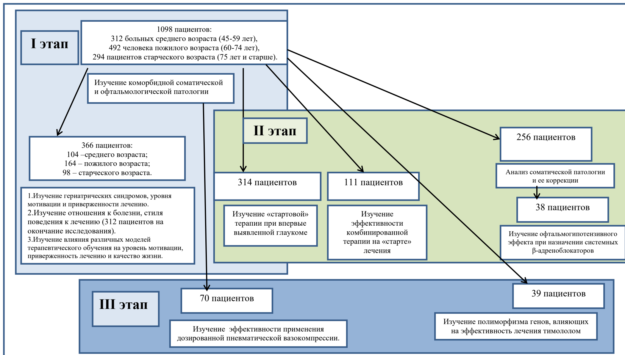
Рис. 1. Дизайн исследования.
